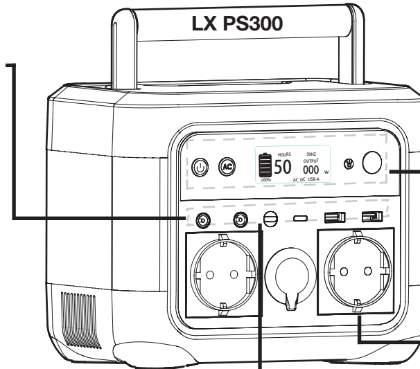
5521 Ladeanschluss
