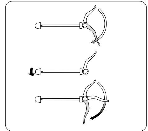
Einstellmutter anziehen
