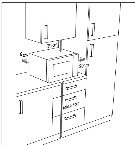
Abb. 2 – Distance entre les appareils
