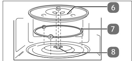
Abb. 3 – Glas-Drehteller einsetzen
