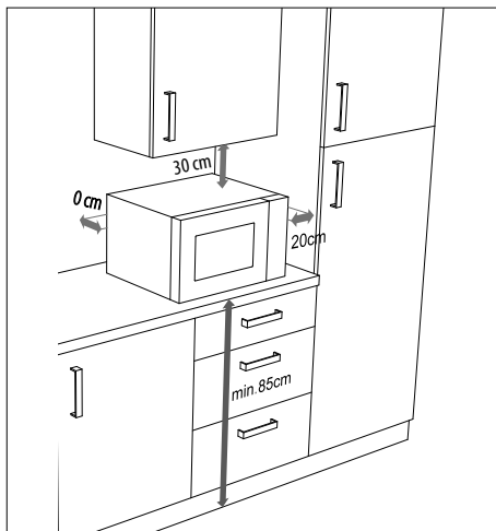
Abb. 2 – Distanza dell'apparecchio
