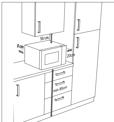
Abb. 2 – Distancias de aparato
